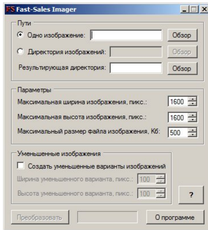
Рис.1. Диалоговое окно программы Fast-Sales Imager
