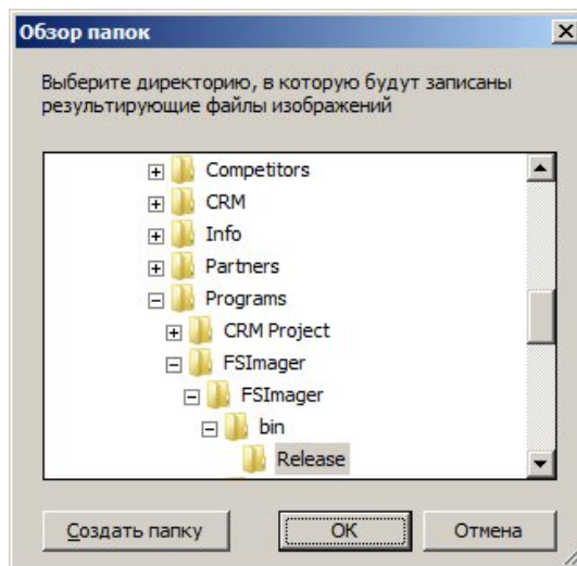
Рис.2. Выбор директории.
