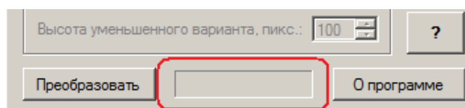
Рис.3. Индикатор прогресса.
